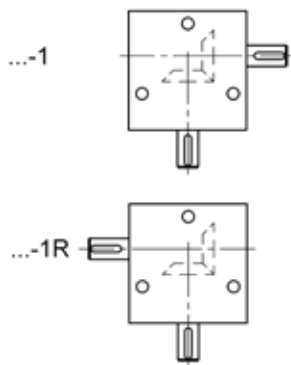
hřídel podle směru otáčení
