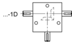
oboustranná výstupní hřídel
